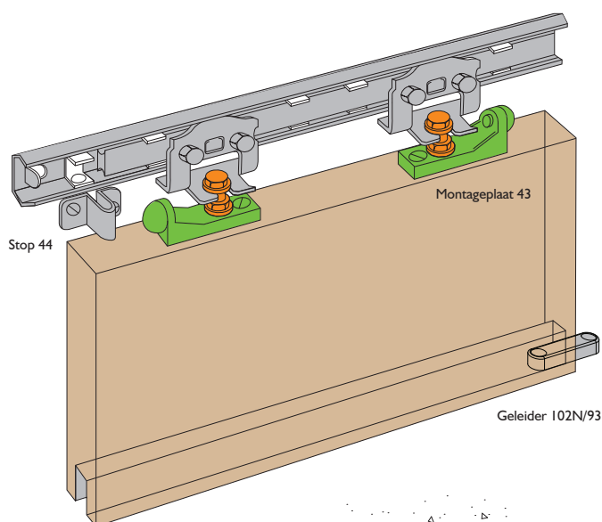
Geleiderail 93S
